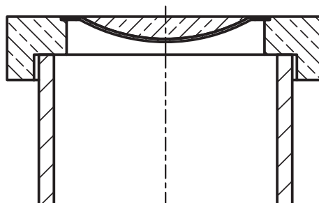
Beton-Guss-Schachtabdeckung Belastungsklasse B (D)
