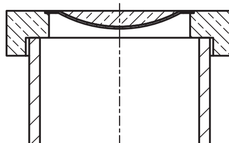
Beton-Guss-Schachtabdeckung Belastungsklasse B (D)
